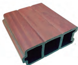
PERFIL DIVISÓRIA 180x73mm PESO: 5,1 Kg/m
